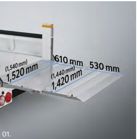
01. 일반형 게이트 규격* ※ ( )는 1.2톤 규격
