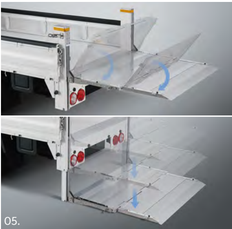
05. 2단 접이식 게이트 개폐 작동*
